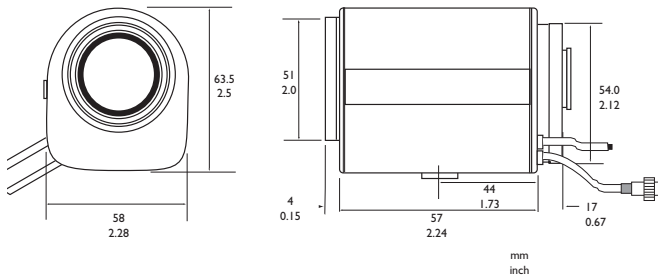
Dimensions LTC 3283/20
